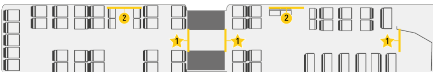
Figur 7 – Illustrasjon av foreslåtte plasseringer av skjermer for ulike busstyper.
