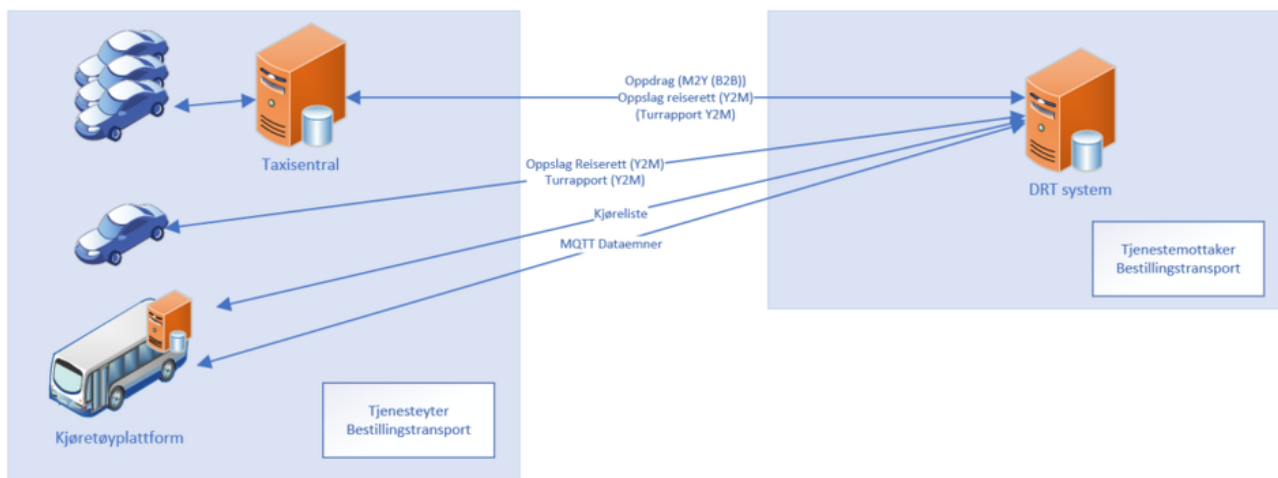
Illustrasjon, eksempler på grensesnitt Tjenestemottaker/Tjenesteyter Bestillingstransport
