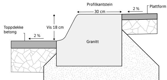
Figur 1.11. Utforming av profilkantstein i granitt ved holdeplass med betongdekke. Betongdekke er mer robust med tanke på slitasje, og gjør det lettere for sjåførene å kjøre helt inn til plattformkant.
