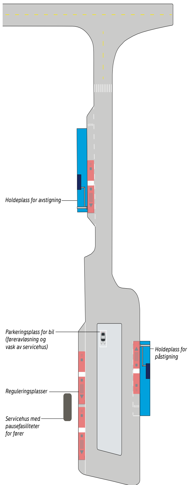
Figur 5.3. Prinsipiell utforming av endeholdeplass med separat reguleringsplass.
