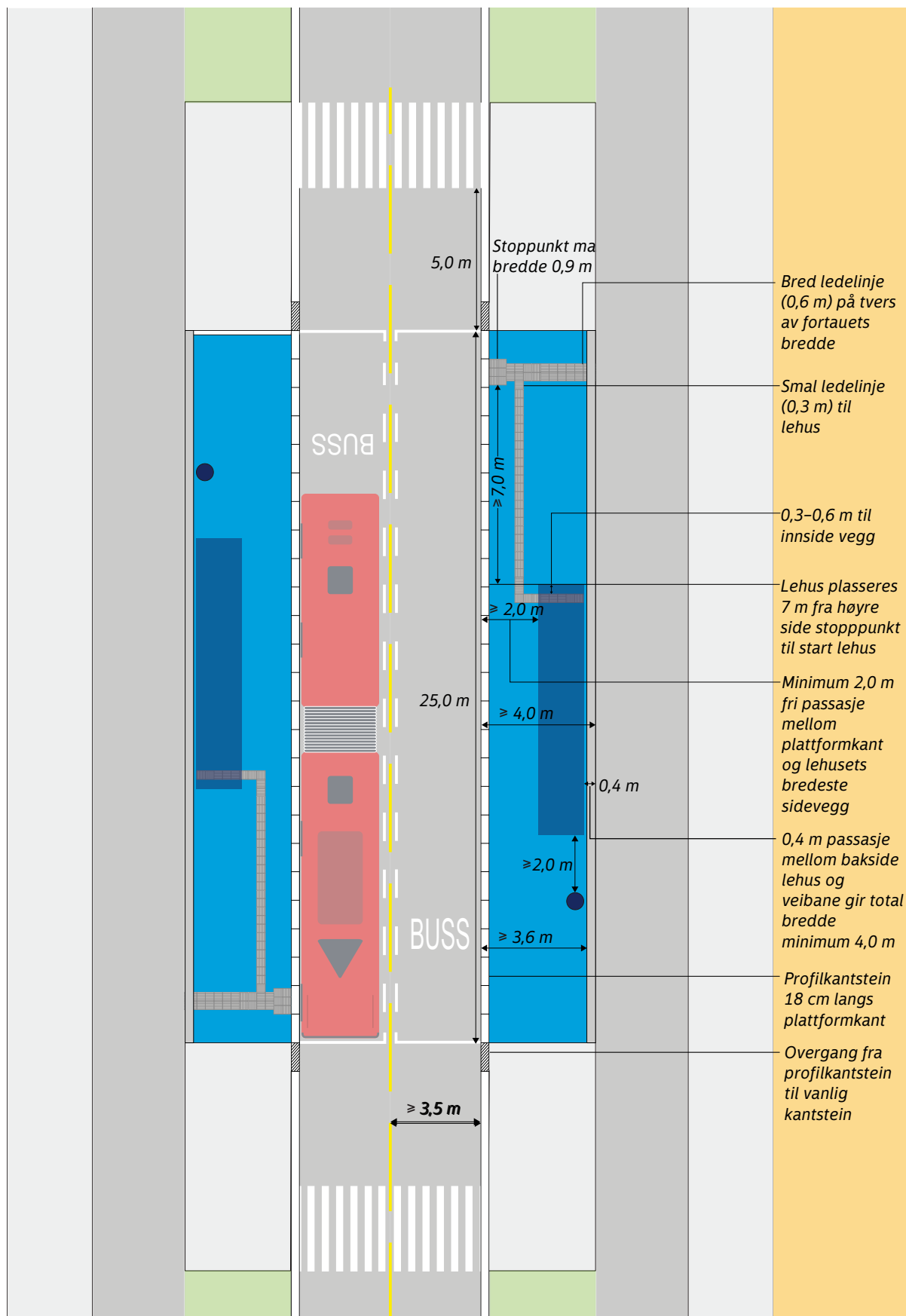
Figur 1.59. Holdeplass ved midtstilt kollektivtrasé. Holdeplassen er vist med seksmoduls lehus. Størrelse på lehus tilpasses etter behov (dimensjonering av lehus er nærmere beskrevet i kapittel 1.3.4). Løsningen er basert på utformingsprinsipper gitt i N-V123 Kollektivveiledning [3]
