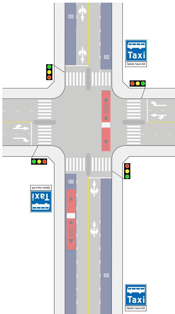
Figur 3.16. Kollektivfelt helt frem til stopplinje – felles kjørefelt for alle svingebevegelser
