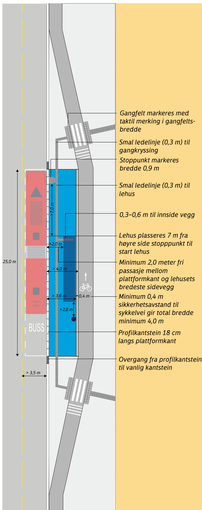
Figur 1.66. Holdeplasser med tilrettelegging for sykkel bak plattform gir et breddebehov på 8,7 meter. Holdeplassen er vist med seksmoduls lehus. Størrelse på lehus tilpasses behov. Dimensjonering av lehus er nærmere beskrevet i kapittel 1.3.4. Løsningen er basert på utformingsprinsipper gitt i N-V123 Kollektivveiledning [3].
