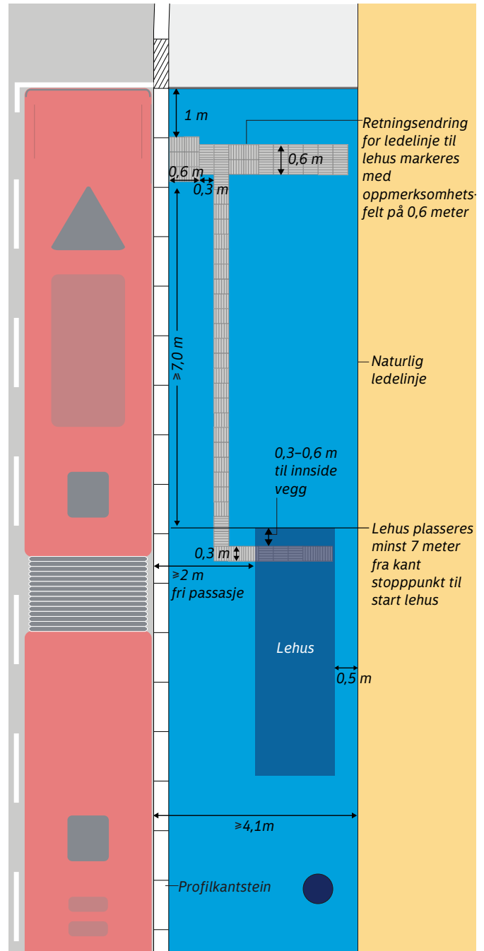
Figur 1.21. Utforming av ledelinje på holdeplass for leddbus med lehus plassert minst 7 meter fra kant stoppunkt til start lehus (standard plassering på holdeplasser som skal kunne betjene leddbus). Ledelinjen på tvers av holdeplassen fanger opp gående langs en vegg (naturlig ledelinje). Det er i tillegg ledelinje fra lehuset til markering av stoppunkt. Dersom naturlig ledelinje er en vegg, skal det være minimum 0,5 meter avstand bak lehus for vedlikehold (som vist på tegningen). Tegningen viser tremoduls lehus. Størrelse på lehus tilpasses behov, se kapittel 1.3.4.
