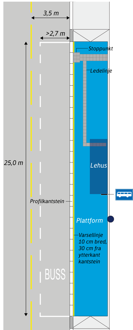
Figur 1.18. Oppmerking ved holdeplass i gate uten parkering. Holdeplassen er vist med tremoduls lehus plassert minst 7 meter fra kant stoppunkt til start lehus (standard plassering på holdeplasser som skal kunne betjene inntil 25 meter lang toleddsbus).
