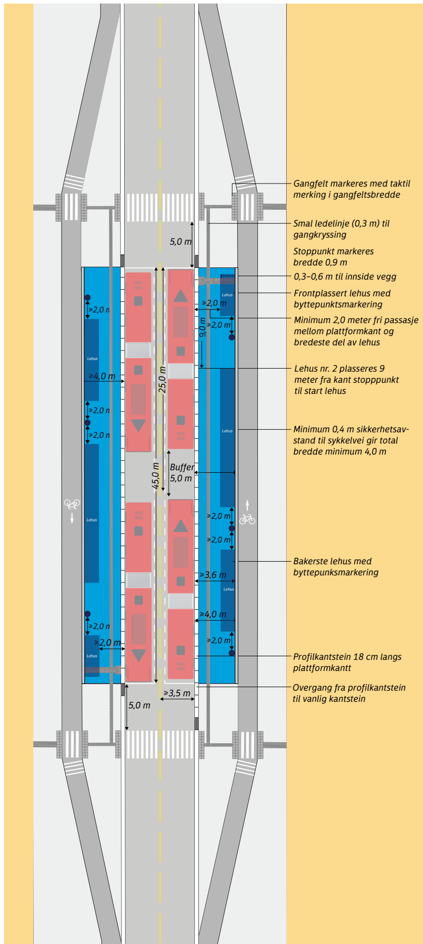
Figur 1.68. Kantstopp i byttepunkt med plass til to leddbusser med tilrettelegging for sykkel bak plattform gir et breddebehov på 8,7 meter. Holdeplassen er vist med et frontplassert tremodulslehus med byttepunktmarkering og et 10 moduls lehus. I tillegg er det en plassert søyle med byttepunktmarkering lengst bak på plattform. Eksemplet er vist med flere Lehus for å vise en situasjon med stort marked. Størrelse på lehus tilpasses behov (dimensjonering av lehus er nærmere beskrevet i kapittel 1.3.4). Illustrasjonen viser en plattform som er bredere enn minimumsmålene. Løsningen er basert på utformingsprinsipper gitt i N-V123 Kollektivveiledning [3].
