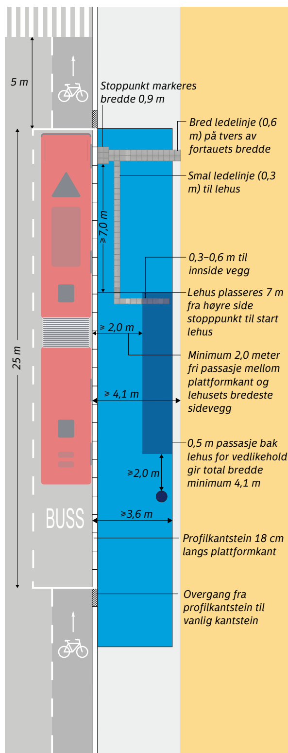
Figur 1.64. Holdeplasser hvor "vanlig" sykkelfelt opphører. Holdeplassen er vist med seksmoduls lehus. Størrelse på lehus tilpasses behov (dimensjonering av lehus er nærmere beskrevet i kapittel 1.3.4). Illustrasjonen viser en plattform som er bredere enn minimumsmålene. Løsningen er basert på utformingsprinsipper gitt i N-V123 Kollektivveiledning [3].
