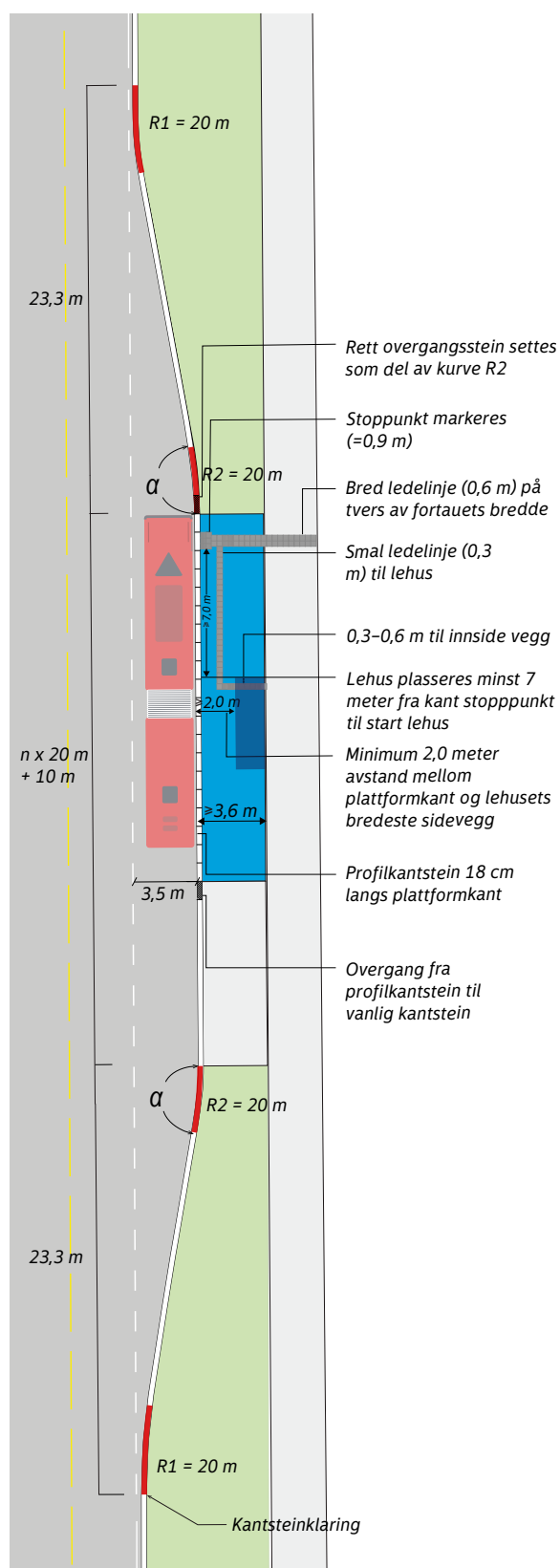
Figur 1.48. Busslomme uten refuge med krav gitt av hastigheter under 80 km/t. For høyere hastigheter, se Tabell 1.4. Vist for hastighet < 80 km/t. Løsningen er basert på utformingsprinsipper gitt i N-V123 Kollektivveiledning [3].
