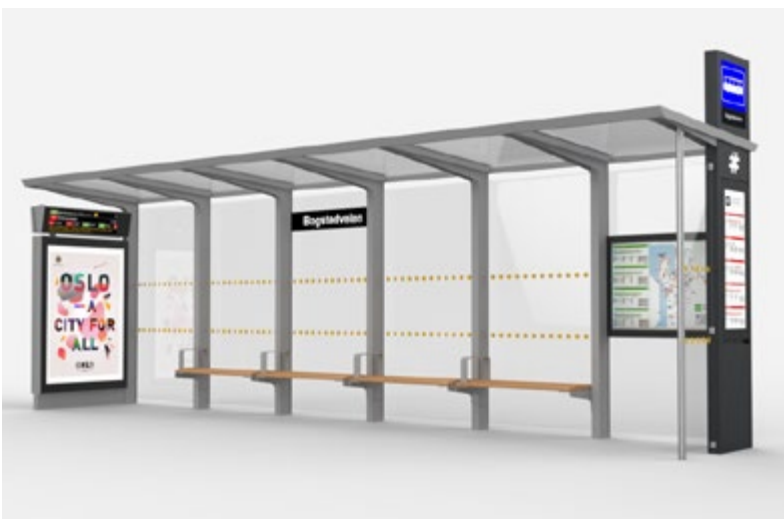
Figur 1.38. Standard seksmoduls lehus med lengde ca. 8,8 meter. Anbefalt brukt ved større kundegrnlag. Illustrasjon: UIP.
