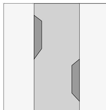
Figur 2.19. Sideforskyvning. Løsningen er hentet fra håndbok V128 Fartsdempende tiltak [8].
