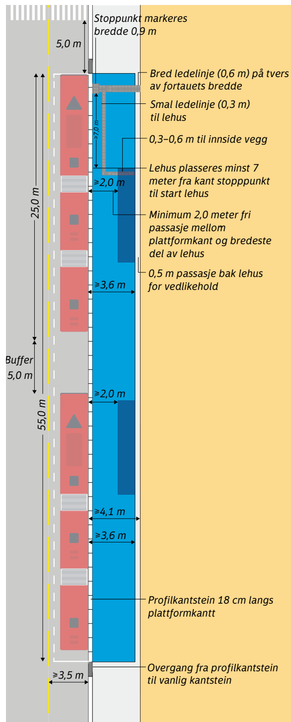
Figur 1.54. Kantstopp med plass til to busser etter hverandre. Holdeplassen er vist med seksmodul lehus. Størrelse på lehus tilpasses behov (dimensjonering av lehus er nærmere beskrevet i kapittel 1.3.4). Illustrasjonen viser en plattform som er bredere enn minimumsmålene. Løsningen er basert på utformingsprinsipper gitt i N-V123 Kollektivveiledning [3].
