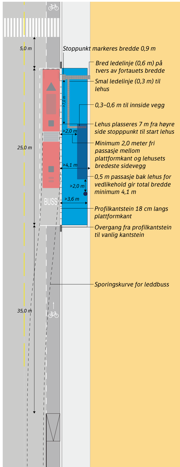
Figur 1.65. Opphøyet sykkelfelt som opphører gjennom holdeplassen. Stiplet linje viser sporingskurve for leddbuss, og viser hvor sykkelfeltet må nedrampes. Holdeplassen er vist med seksmoduls lehus. Størrelse på lehus tilpasses behov (dimensjonering av lehus er nærmere beskrevet i kapittel 1.3.4). Illustrasjonen viser en plattform som er bredere enn minimumsmålene.
