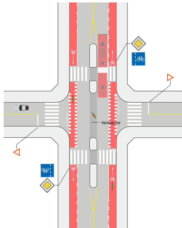
Figur 3.24. Forkjørsregulert tofelts kryss med gjennomgående sykkel felt og ventesone for venstresvingende syklist.
