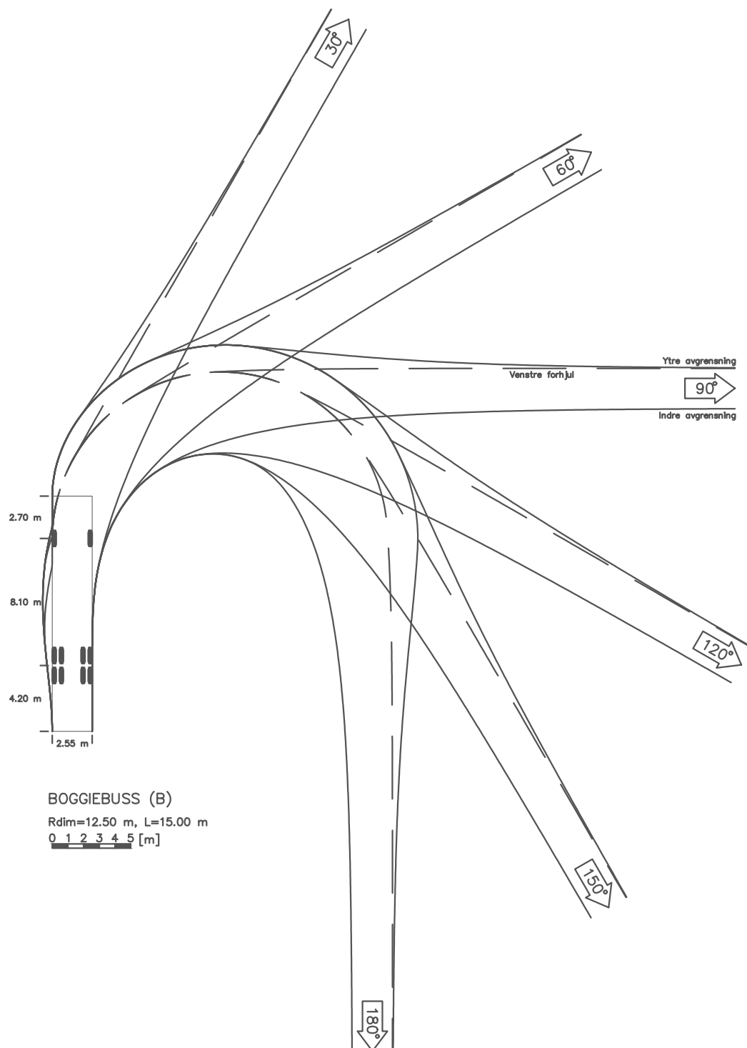
Figur 6.1. Sporingkurver for dimensjonerte buss (boggiebus).
