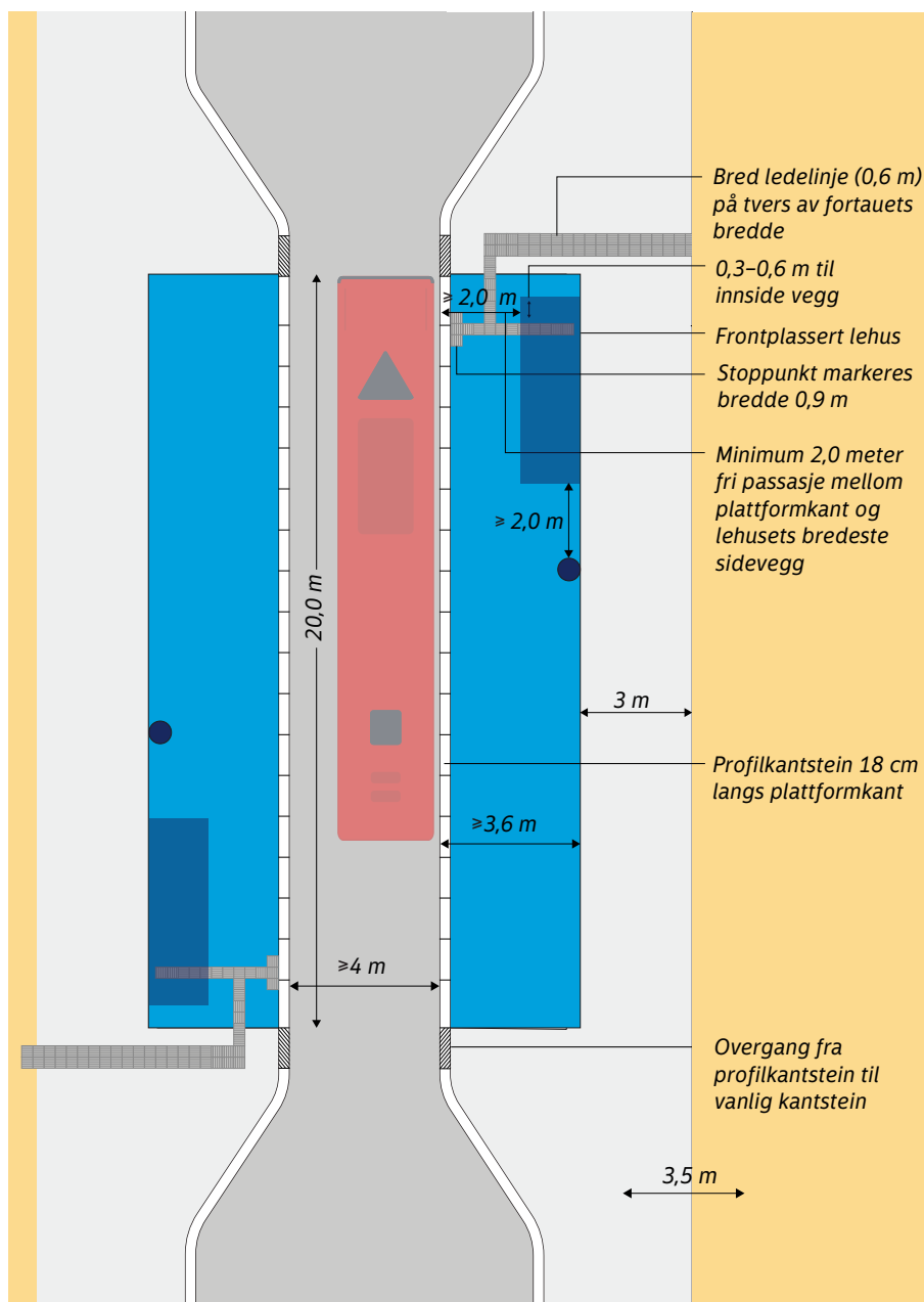
Figur 1.60. Holdeplass med timeglassutforming. Holdeplassen er vist med tremodul lehus. Størrelse på lehus tilpasses behov (dimensjonering av lehus er nærmere beskrevet i kapittel 1.3.4). Illustrasjonen viser plattformer som er bredere enn minimumsmålene. Løsningen er basert på utformingsprinsipper gitt i N-V123 Kollektivveiledning [3].
