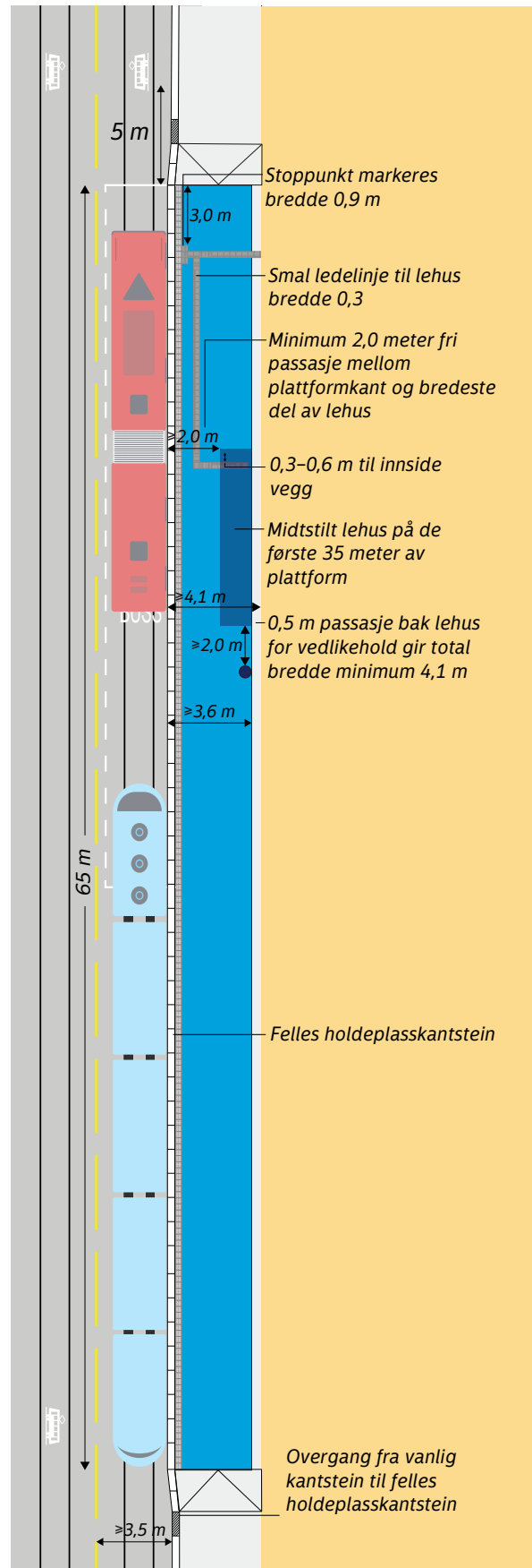
Figur 1.62. Felles holdeplass for buss og trikk, med felles kantstein. Holdeplassen er vist med seksmodulslehus. Størrelse på lehus tilpasses behov (dimensjonering av lehus er nærmere beskrevet i kapittel 1.3.4). Illustrasjonen viser en plattform som er bredere enn minimumsmålene.
