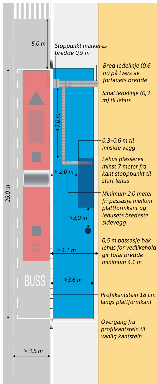
Figur 1.50. Kantstopp. Denne løsningen krever at man har en kjørefeltbredde på minimum 3,5 meter. Holdeplassen er vist med tremodus lehus. Størrelse på lehus tilpasses behov (dimensjonering av lehus er nærmere beskrevet i kapittel 1.3.4). Illustrasjonen viser en plattform som er bredere enn minimumsmålene. Løsningen er basert på utformingsprinsipper gitt i N-V123 Kollektivveiledning [3].
