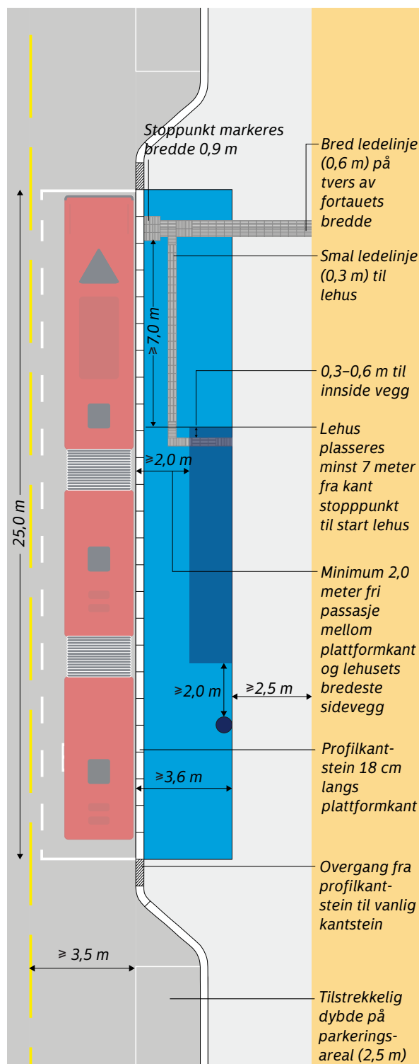
Figur 1.53. Kantstopp med utlagt plattform. Holdeplassen er vist med seksmoduls lehus. Størrelse på lehus tilpasses behov (dimensjonering av lehus er nærmere beskrevet i kapittel 1.3.4). Løsningen er basert på utformingsprinsipper gitt i N-V123 Kollektivveiledning [3].
