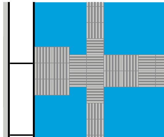
Figur 1.67. Utforming av stoppunkt ved frontplassert lehus og leding til gangfelt over sykkelkjørebane og sykkelfelt eller sykkelvei.
