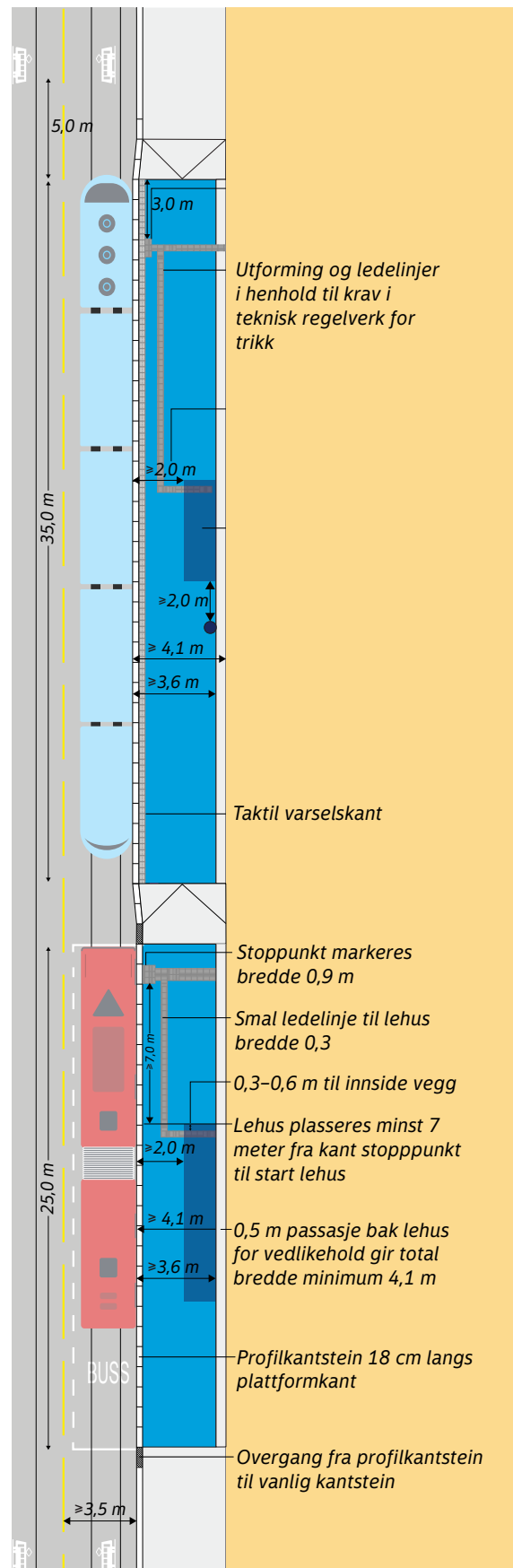
Figur 1.63. Felles holdeplass for buss og trikk, med stoppested på hver sin del av plattformen. Holdeplassen er vist med tremoduls lehus. Størrelse på lehus tilpasses behov (dimensjonering av lehus er nærmere beskrevet i kapittel 1.3.4). Illustrasjonen viser plattformer som er bredere enn minimumsmålene.
