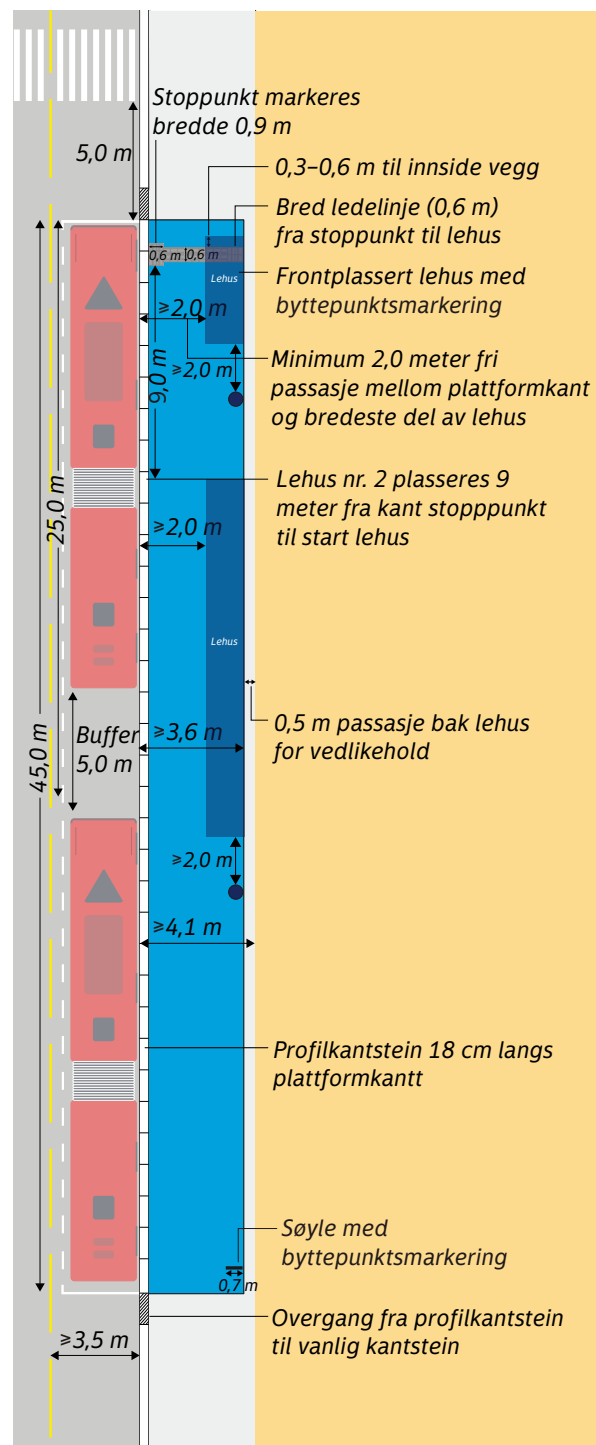
Figur 1.55. Kantstopp i byttepunkt med plass til to leddbusser. Holdeplassen er vist med et frontplassert tremodulslehus med puck og et 10 moduls lehus. I tillegg er det plassert søyle med byttepunktmarkering lengst bak på plattform. Størrelse på lehus tilpasses behov (dimensjonering av lehus er nærmere beskrevet i kapittel 1.3.4). Illustrasjonen viser en plattform som er bredere enn minimumsmålene. Løsningen er basert på utformingsprinsipper gitt i N-V123 Kollektivveiledning [3].
