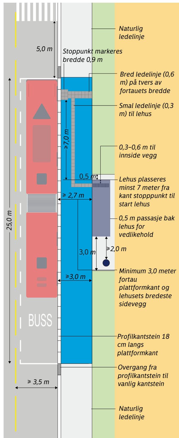
Figur 1.51. Kantstopp med lehus bak plattform. Denne løsningen krever at man har en kjørefeltbredde på minimum 3,5 meter. Holdeplassen er vist med tremoduls lehus. Størrelse på lehus tilpasses behov (dimensjonering av lehus er nærmere beskrevet i kapittel 1.3.4). Løsningen er basert på utformingsprinsipper gitt i N-V123 Kollektivveiledning [3].
