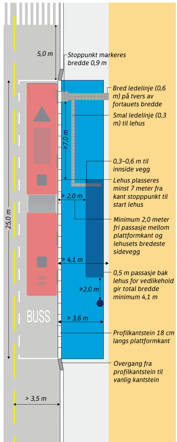
Figur 1.52. Kantstopp med delvis utlagt plattform. Denne løsningen krever at man har en kjørefeltbredde på minimum 3,5 meter. Holdeplassen er vist med seksmodul lehus. Størrelse på lehus tilpasses behov (dimensjonering av lehus er nærmere beskrevet i kapittel 1.3.4). Illustrasjonen viser en plattform som er bredere enn minimumsmålene.
