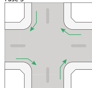
Figur 3.11. Signalveksling med 3 faser
