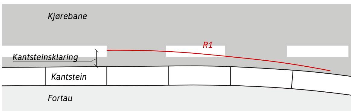
Figur 1.47. Busslomme detalj av radius R1 ved inn- og utkjøring. Radius R1 viser til kurve ved innkjøring og utkjøring fra busslomme, (se Figur 1.48).
