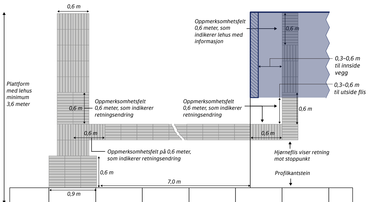
Figur 1.20. Detaljerte prinsipper for utforming av ledlinjer mellom lehus og stoppunkt, for midtplassert lehus. Hovedprinsippene er basert på N-V123 Kollektivveiledning [3].
