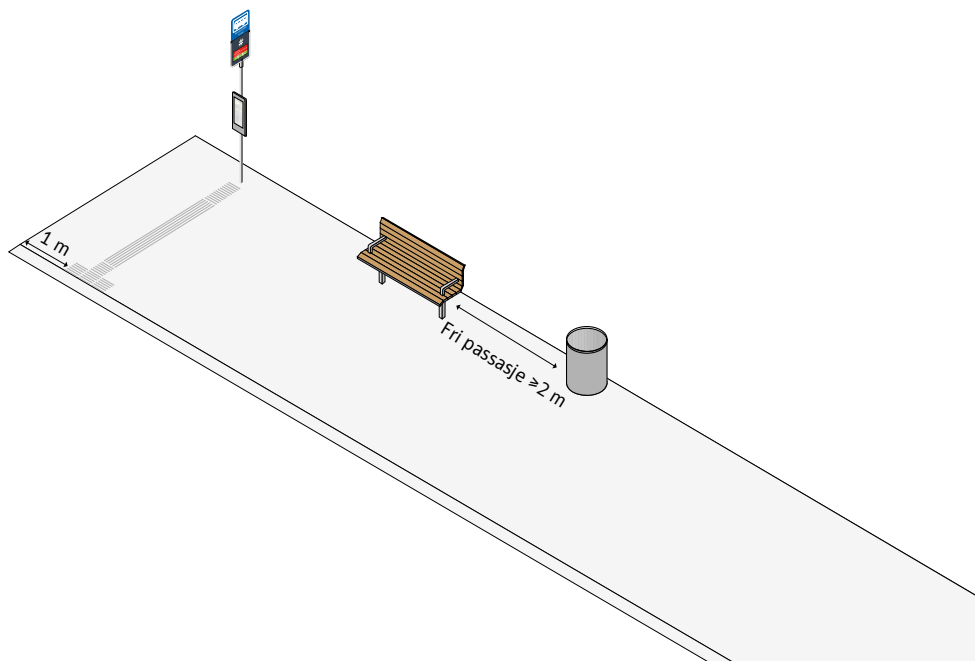
Figur 1.33. Standard holdeplass med toppskilt
