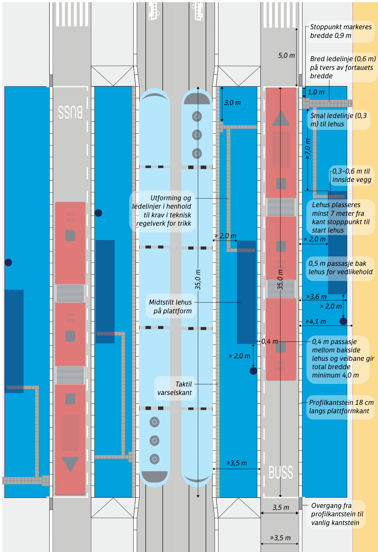
Figur 1.61. Felles holdeplass for buss og trikk med parallelle oppstillingsplasser. Merk at trikkeholdeplass utformes etter krav i Teknisk regelverk for byspor/forstadsbaner [14]. Dette innebærer blant annet 35 meter lang plattform med midtstilt lehus og taktil varselkant langs hele plattformen. Bussholdeplass kan forlenges slik at den blir like lang som trikkeholdeplassen og utformes for øvrig som vanlig kantstopp. Holdeplassen er vist med seksmoduls lehus. Størrelse på lehus tilpasses etter behov (dimensjonering av lehus er nærmere beskrevet i kapittel 1.3.4). Illustrasjonen viser plattformer for buss som er bredere enn minimumsmålene.
