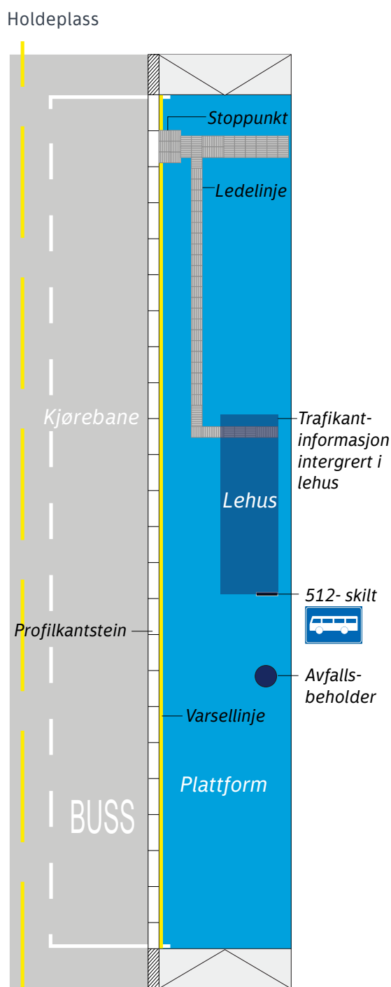
Figur 1.1. Elementer på en holdeplass. Holdeplassen er vist med tremoduls lehus plassert minst 7 meter fra kant stoppunkt til start lehus (standard plassering på holdeplasser som skal kunne betjene leddbuss). Plassering (frontplassert eller "midtplassert") og størrelse på Lehus tilpasses behov, se kapittel 1.3.4.
