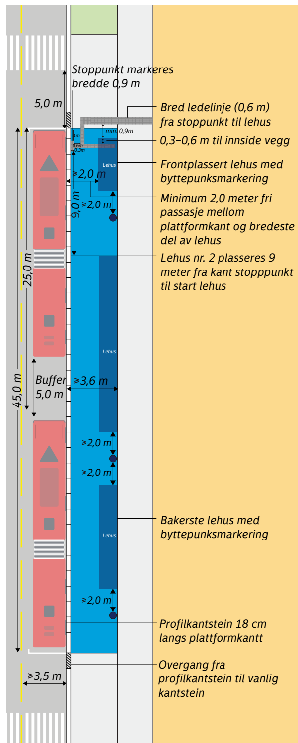
Figur 1.56. Kantstopp i byttepunkt med plass til to leddbusser med fortau bak plattform. Holdeplassen er vist med et frontplassert tremodul lehus med byttepunktmarkering og et 10 moduls lehus. I tillegg er den vist med et tredje lehus med stoppunktmarkering i stedet for søyle lengst bak på plattform. Eksemplet er vist med flere Lehus for å vise en situasjon med stort marked. Størrelse på lehus tilpasses behov (dimensjonering av lehus er nærmere beskrevet i kapittel 1.3.4). Illustrasjonen viser en plattform som er bredere enn minimumsmålene. Løsningen er basert på utformingsprinsipper gitt i N-V123 Kollektivveiledning [3].
